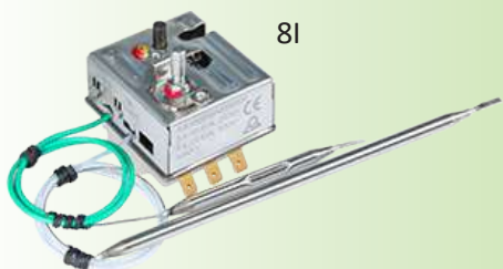
Однополюсный термостат высокого предела с ручным сбросом, отказоустойчивый, фиксированная настройка, диапазон температур до 320°C
