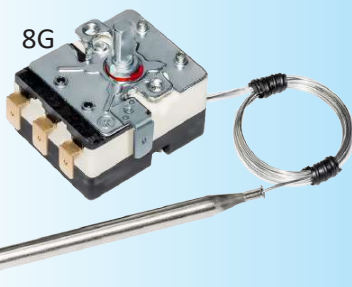
Однополюсный патронный и капиллярный термостат, диапазон температур до 500°C
